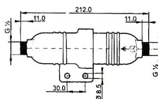
COD. 19044 FILTRO SILURO OTTONE CON CARTUCCIA INOX
