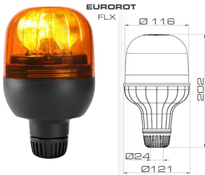
FARO ROTANTE EUROROT SIRENA CON SUPPORTO ELASTICO Cod. 08185
