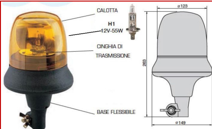
FARO ROTANTE COBO PICCOLO CON SUPPORTO ELASTICO Cod. 08195
