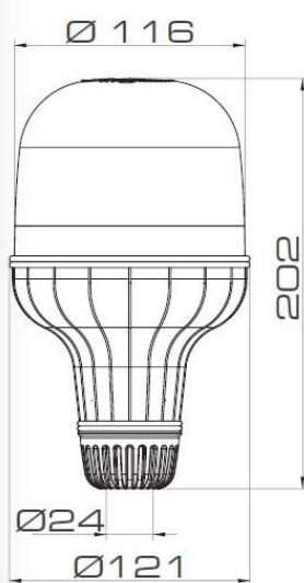
FARO ROTANTE EUROROT SIRENA CON SUPPORTO ELASTICO Cod. 08185
