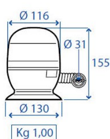
FARO ROTANTE SACEX RIBASSATO 12/24 V BASE MAGNETICA Cod. 08179
