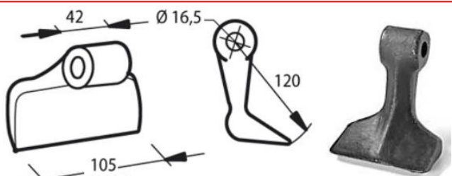
Cod. 18063 MAZZA RM47 (FERRI LEGGERA) foro mm 16,5
