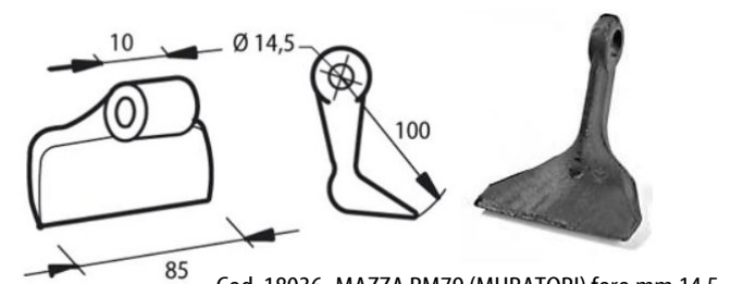
Cod. 18036 MAZZA RM79 (MURATORI) foro mm 14,5
