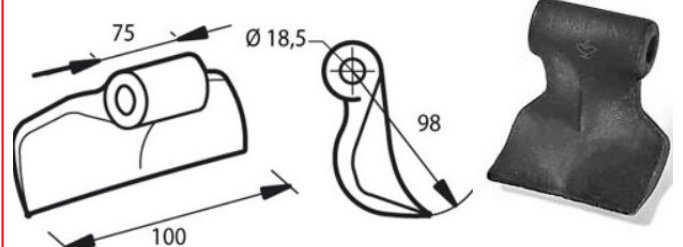
Cod. 18061 MAZZA RM36 (DRAGONE) foro mm 18,5
