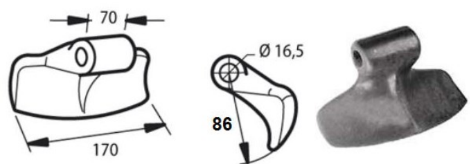
Cod. 18039 MAZZA RM31 (HMF-PALLADINO) foro mm 16,5
