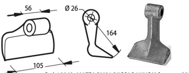
Cod. 18068 MAZZA RM91 (VIGOLO LUNGA) foro mm 25,5
