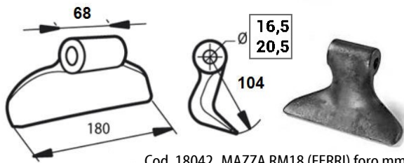
Cod. 18042 MAZZA RM18 (FERRI) foro mm 16,5 Cod. 18045 MAZZA RM18 (FERRI) foro mm 20,5
