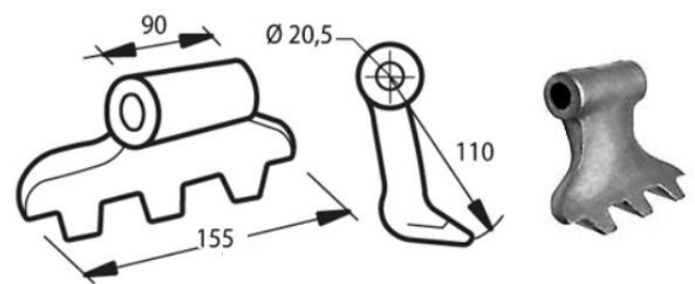
Cod. 18069 MAZZA RM2 (NOBILI DENTELLATA) foro mm 20,5
