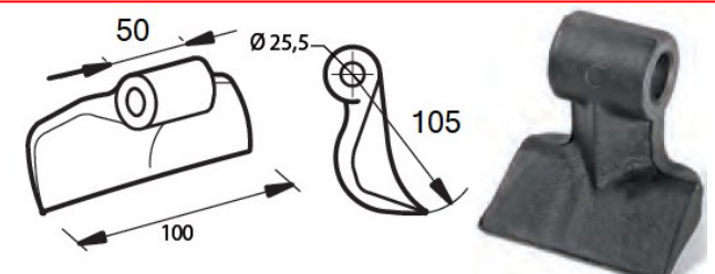
Cod. 18067 MAZZA RM40 (NOBILI MEDIA) foro mm 25,5
