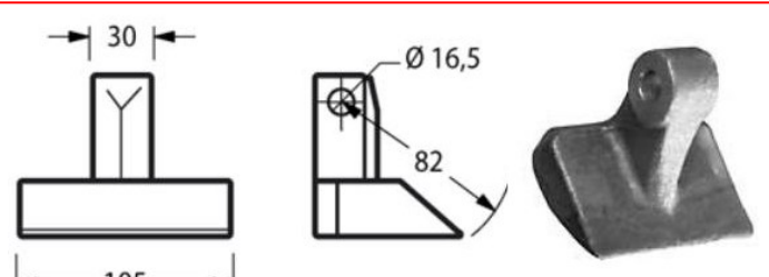
Cod. 18065 MAZZA MER06 (MERITANO) foro mm 16,5
