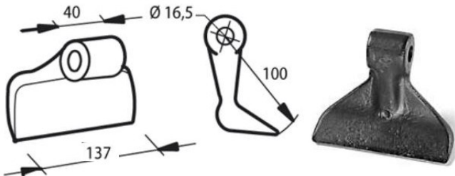
Cod. 18054 MAZZA RM30 (BERTI LEGGERA) foro mm 16,5
