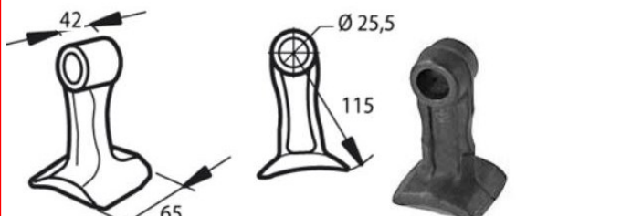
Cod. 18048 MAZZA RM20 (FERRI PICCOLA) foro mm 25,5
