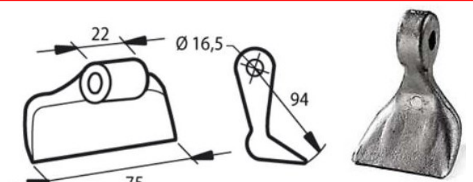
Cod. 18051 MAZZA RM32 (VIGOLO) foro mm 16,5
