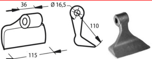
Cod. 18066 MAZZA RM43 (NOBILI LEGGERA) foro mm 16,5
