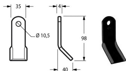
Cod. COLTELLO DECESP. ZAPPATOR 35x4x98 F. 17687 10,5 {ZAP12}
