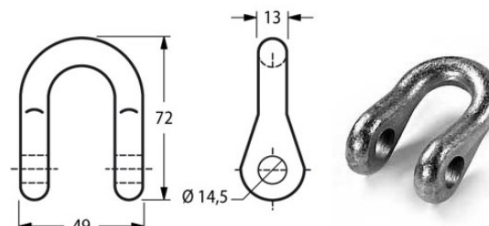
Cod. 17944 CAVALLOTTO MAROLIN (FILO 13 FORO 14,5)
