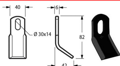
Cod. COLTELLO DECESP. FERRI A "Y" ASOLA 17553 40x6x82 F. 30x14 {FEI57}
