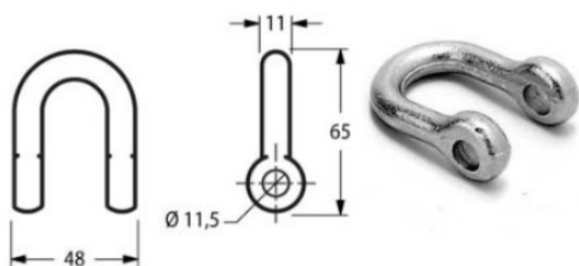
Cod. 17901 CAVALLOTTO HYMAC (E ALTRI) FORO 11,5
