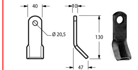
Cod. COLTELLO DECESP. MEAAT 40x10 f. 20,5 17591 {MEA11}
