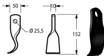
Cod. COLTELLO DECESP. ORSI GIRATO 50x10 Ø 25 17633 {ORS04}
