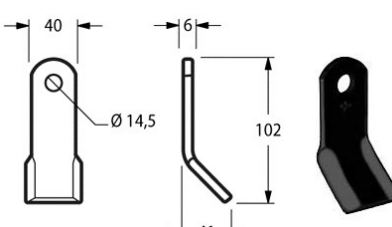
Cod. COLTELLO DECESP. ZAPPATOR 40x6x102 F. 17688 14,5 {ZAP13}
