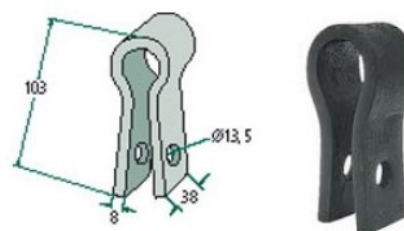
Cod. 17934 CAVALLOTTO TAARUP
