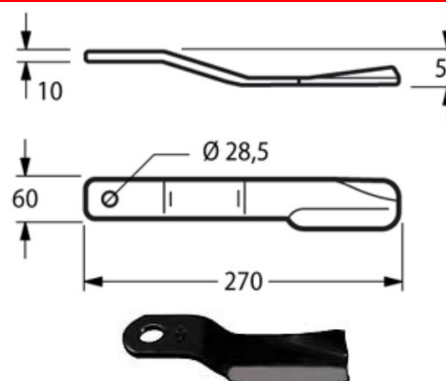
Cod. 17965 COLTELLO RASAERBA FISCHER mm 70 {VIG07}
