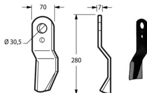
Cod. 17966 COLTELLO RASAERBA OMMAS 70x7 {OMM02}
