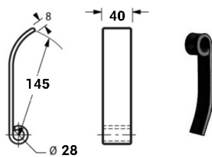
Cod. 17857 COLTELLO RICCIO VIGOLO 40x8 Ø 28,5 {VIG04}
