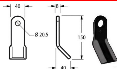
Cod. COLTELLO DECESP. ORSI RIVER 500 40x8 F. 17636 20,5 {ORS12}
