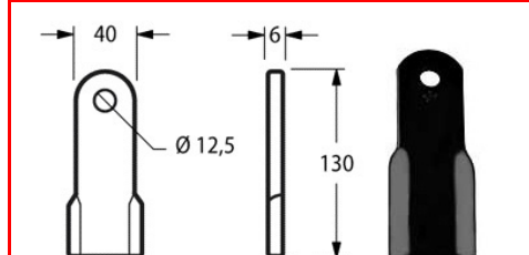
Cod. COLTELLO DECESP. FERRI DIRITTO 40x6x130 17552 F. Ø 12 {FEI55}
