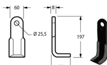
Cod. 17820 COLTELLO TRINCIASTOCCHI SICMA 60x8 90° {SIC03}
