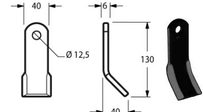
Cod. COLTELLO DECESP. FERRI A "Y" 40x6x130 F. Ø 17551 12 {FEI54}
