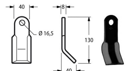
Cod. COLTELLO DECESP. FERRI 40x8x127 F. Ø 16,5 17550 'TIP' {FEI45}
