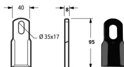
Cod. COLTELLO DECESP. MAROLIN-ORSI DIRITTI 40x8 17589
