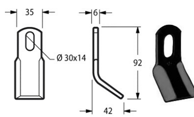
Cod. COLTELLO DECESP. NOBILI BNE08 35x6 17626 {NOB35}
