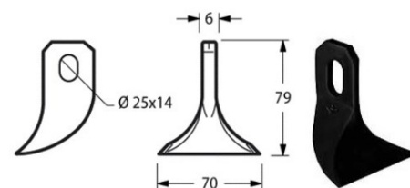
Cod. COLTELLO DECESP. SOVEMA SPATOLA 70x3 17686 {SOV19}
