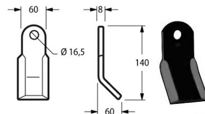
Cod. COLTELLO DECESP. ORSI 60x8 F. 16,5 {ORS01} 17635
