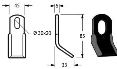
Cod. COLTELLO DECESP. SEPPI 45x6 {SPI04} 17662
