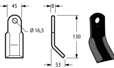
Cod. COLTELLO DECESP. NOBILI VKD210 45x8 17625 {NOB27}
