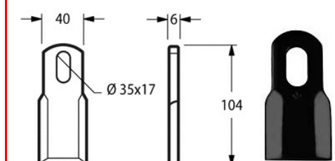
Cod. COLTELLO DECESP. FERRI 40x8x100 AS.35x17 17549 DIRITTO {FEI49}
