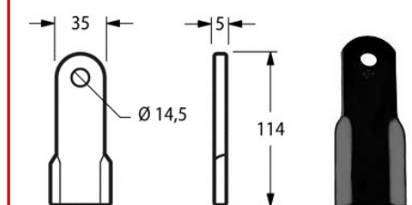
Cod. COLTELLO DECESP. MURATORI DIR. 35x5 f.15 17594 {MUR22}
