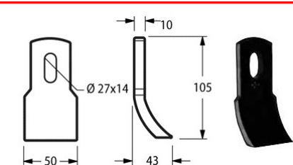
Cod. COLTELLO DECESP. HYMAC PALETTA 17568 50x10x105 AS. 27x14 {HYM10}
