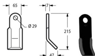
Cod. 17840 COLTELLO TRINCIASTOCCHI TAARUP 65x7 {TAA02}
