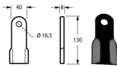
Cod. COLTELLO DECESP. NOBILI-FERRI DIRITTO 17629 40x8x130 {NOB17}
