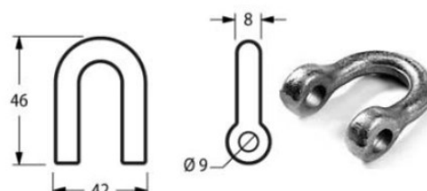
Cod. 17940 CAVALLOTTO HERMES-TERRANOVA 42x46 FORO 8,5
