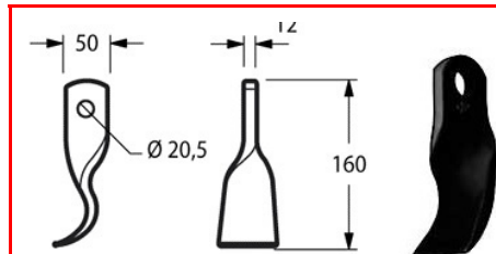
Cod. COLTELLO DECESP. HYMAC GIRATO 50x12 17570 {HYM12}
