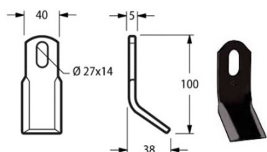
Cod. COLTELLO DECESP. SMA LUNGO 40x5 17680 {ROU02}
