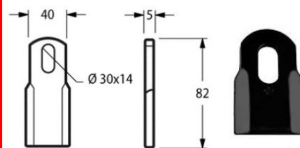
Cod. COLTELLO DECESP. SMA CORTO DIRITTO 40x5 17672 {S.MO04}
