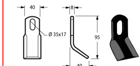
Cod. COLTELLO DECESP. MAROLIN-ORSI 45° 40x8 17588 {ORS06}
