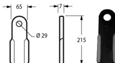
Cod. 17850 COLTELLO TRINCIASTOCCHI TAARUP 65x7 DIRITTO {TAA01}
