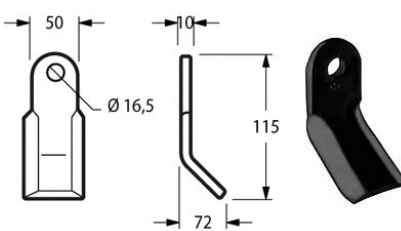
Cod. COLTELLO DECESP. MEAAT 50x10 f. 16,5 17592 {MEA10}
