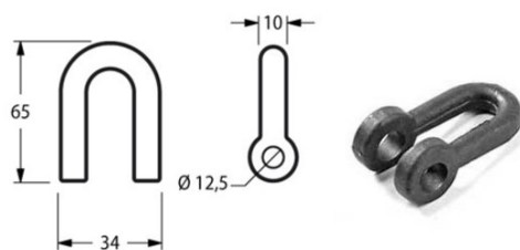
Cod. 17943 CAVALLOTTO MALETTI STRETTO
