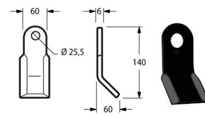
Cod. COLTELLO DECESP. PROCOMAS 60x6 {PRO01} 17660
