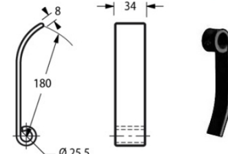
Cod. 17952 PALETTA VENTILANTE NOBILI BMG 34x8 {VIG05}
