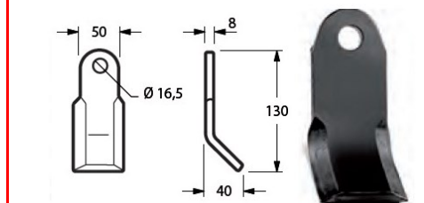
Cod. COLTELLO DECESP. FERRI 50x8x130 h40 F. Ø 17556 16,5 {579CL-FEI60}
