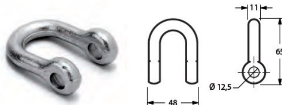
Cod. 17902 CAVALLOTTO FERRI (E ALTRI) FORO 12,5
