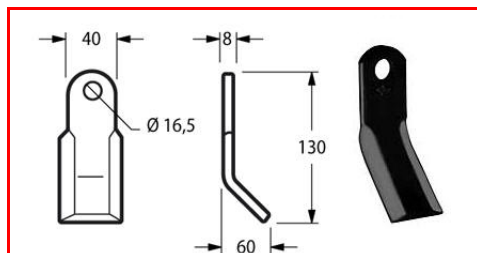
Cod. COLTELLO DECESP. FERRI 40x8 POLIVALENTE 17546 {FEI34}
