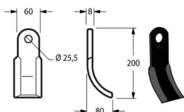
Cod. 17856 COLTELLO TRINCIASTOCCHI VIGOLO 60x8 Ø 25 L 200 H 80 {VIG03}
