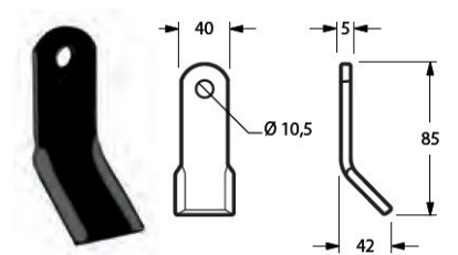
Cod. COLTELLO DECESP. HYMAC-MORELLATO 40x5 17563 F. 10,5 {150025}
