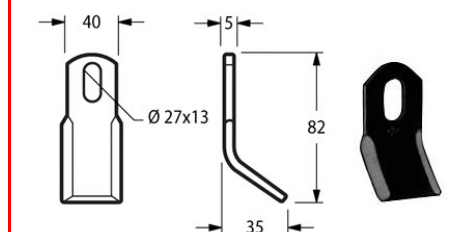
Cod. COLTELLO DECESP. MALETTI FM SASSI 40x5 17585 {MAL24}
