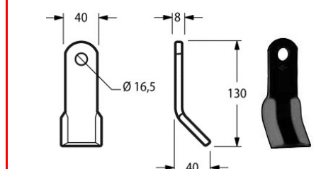
Cod. COLTELLO DECESP. NOBILI BNE 40x8 {NOB16} 17620
