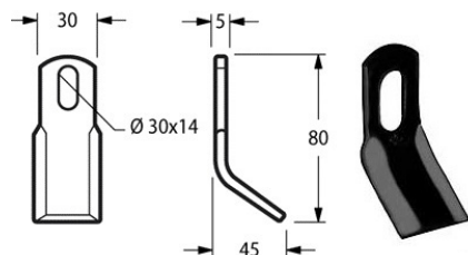
Cod. COLTELLO DECESP. PROCOMAS 30x5 {PRO06} 17640
