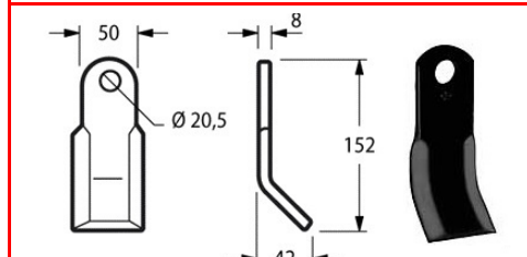
Cod. COLTELLO DECESP. HYMAC 50x8 F. 20,5 17566 {HYM02}
