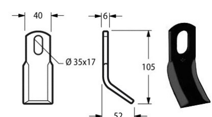
Cod. COLTELLO DECESP. GIMAC 40x6 {GIM03} 17560
