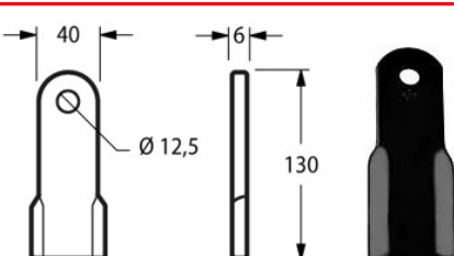
Cod. COLTELLO DECESP. HYMAC 50x8 F. 20,5 L 145 17567 DIRITTO
