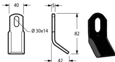
Cod. COLTELLO DECESP. SMA CORTO 40x5 17670 {S.MO01}
