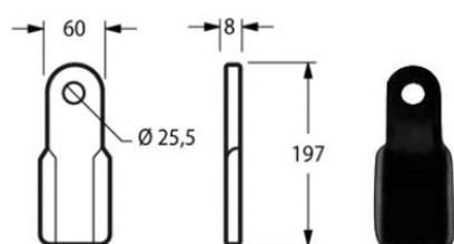
Cod. 17815 COLTELLO TRINCIASTOCCHI SICMA 60x8 DIRITTO {SIC04}
