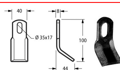
Cod. COLTELLO DECESP. FERRI 40x8x100 AS.35x17 17548 45° {FEI47}
