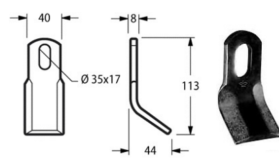
Cod. COLTELLO DECESP. MORIS 40x8 AS. 35x17 L 113 {MRS01}
