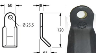
Cod. COLTELLO DECESP. VIGOLO 60X8 Ø 25 L120 H 17702 70
