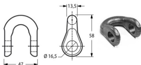
Cod. 17938 CAVALLOTTO BOMFORT FORO Ø mm 16{BOM04}
