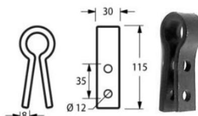
Cod. 17946 CAVALLOTTO NICOLAS 2 FORI
