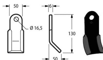
Cod. COLTELLO DECESP. HUMUS 50x6 F. 16,5 17575 {HUM01}
