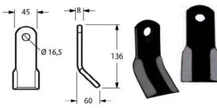
Cod. COLTELLO DECESP. MASCHIO 45x8x136 Ø 16,5 - 45° E DIRITTO {MAS55-MAS58}
