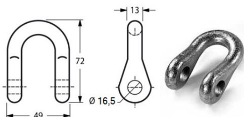
Cod. 17945 CAVALLOTTO ORSI (FILO 13 FORO 16,5)
