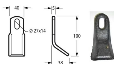
Cod. COLTELLO DECESP. SMA 40x8 {S.MO02} 17685
