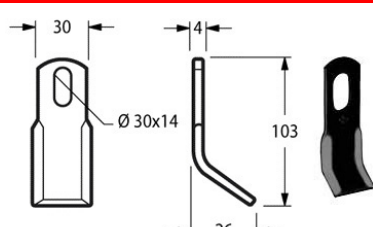
Cod. COLTELLO DECESP. PERUZZO 30x4 {PRZ01} 17637
