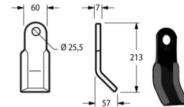
Cod. 17855 COLTELLO TRINCIASTOCCHI TIERRE 60x7 Ø 25 L 220 {TIE03}
