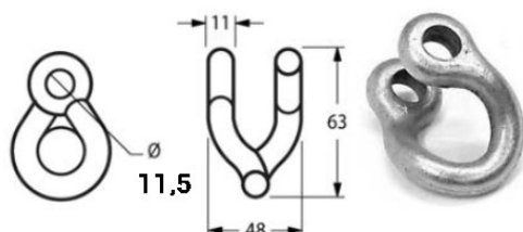
Cod. 17903 CAVALLOTTO RITORTO FORO 11,5
