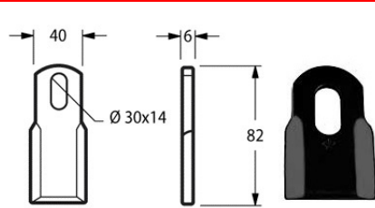
Cod. COLTELLO DECESP. FERRI DIRITTO ASOLA 17554 40x6x82 F. 30x14 {FEI58}
