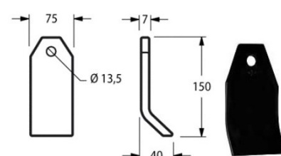
Cod. 17830 COLTELLO TRINCIASTOCCHI TAARUP A PALETTA {TAA03}
