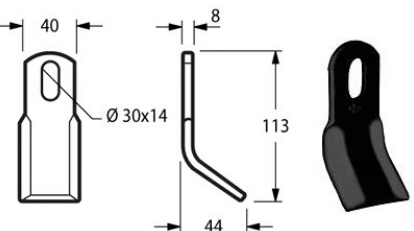
Cod. COLTELLO DECESP. HYMAC 40x8 {HYM01} 17565
