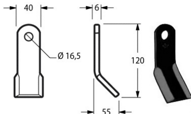
Cod. COLTELLO DECESP. PROCOMAS 40x6 {PRO02} 17650
