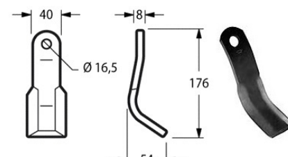
Cod. COLTELLO DECESP. NOBILI BNT 40x8 {NOB02} 17600
