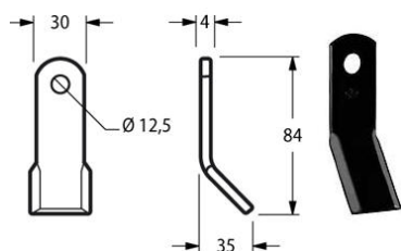
Cod. COLTELLO DECESP. BCS Y 30x4 L 84 Ø 12,5 17661 {BCS20}
