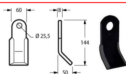
Cod. COLTELLO DECESP. FERRI 60x8 TS CURVO 17547 {FEI51}
