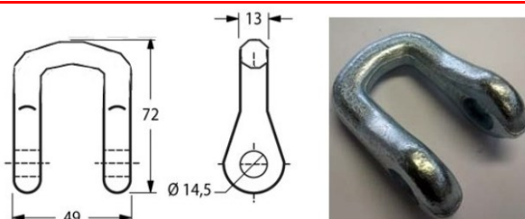
Cod. 17905 CAVALLOTTO E.G.-ROUSSEAU FORO 14,5
