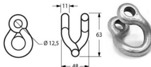
Cod. 17904 CAVALLOTTO FERRI RITORTO FORO 12,5
