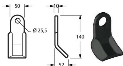
Cod. COLTELLO DECESP. OMARV 50x10 {OMA06} 17631
