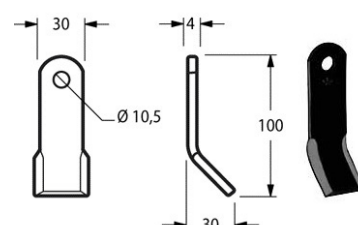
Cod. COLTELLO DECESP. OREC 30x4 f. 10,5 {ORE01} 17630
