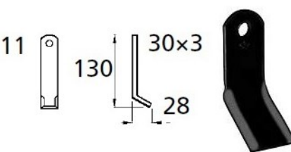
Cod. COLTELLO DECESP. MALETTI FL 30x3x115 17586
