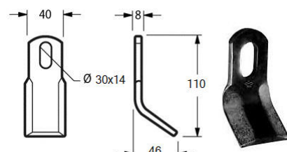
Cod. COLTELLO DECESP. BECCHIO 40X8X110 AS. 17703 30X14
