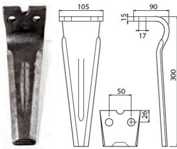
Cod. 06355 - FORIGO-ROTERTALIA 105x15x300 INT. 50
