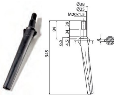
Cod. 06360 - FORIGO CILINDRICO
