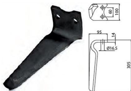
Cod. (Dx/Sx) 06560 - PEGORARO 100x14x305 INT. 60 (CON LUNETTA)
