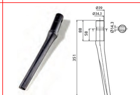
Cod. 06320 - FERABOLI FS A SPINA Ø 34
