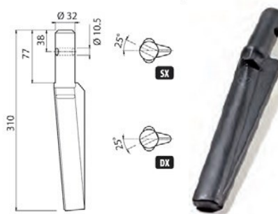
Cod. 06230 - BREVIGLIERI CILINDRICO Dx-Sx TB/333
