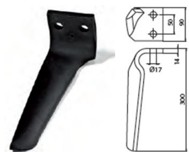
Cod. (Dx/Sx) 06453 - MASCHIO DIAMANTE PESANTE 90x14x300 LUNGO
