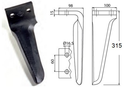
Cod. (Dx/Sx) 06462 - MASCHIO DOMINATOR 100x15x315 INT. 60 (DM-AQUILA RINFORZATO)
