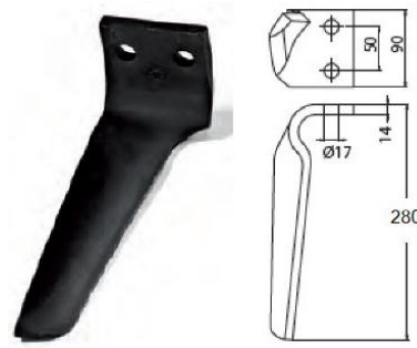
Cod. (Dx/Sx) 06452 - MASCHIO DIAMANTE PESANTE 90x14x280
