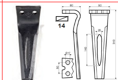
Cod. 06350 - FORIGO-ROTERTALIA 90x14x290 INT. 50
