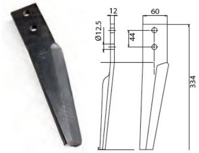
Cod. (Dx/Sx) 06430 - MASCHIO ROTOTERRA HB RINFORZATO 60x12x334
