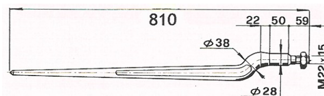
DENTE mm 38x810 DISASSATO
